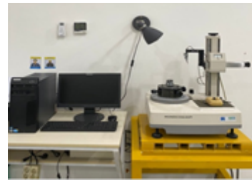
Rondcomp Test
